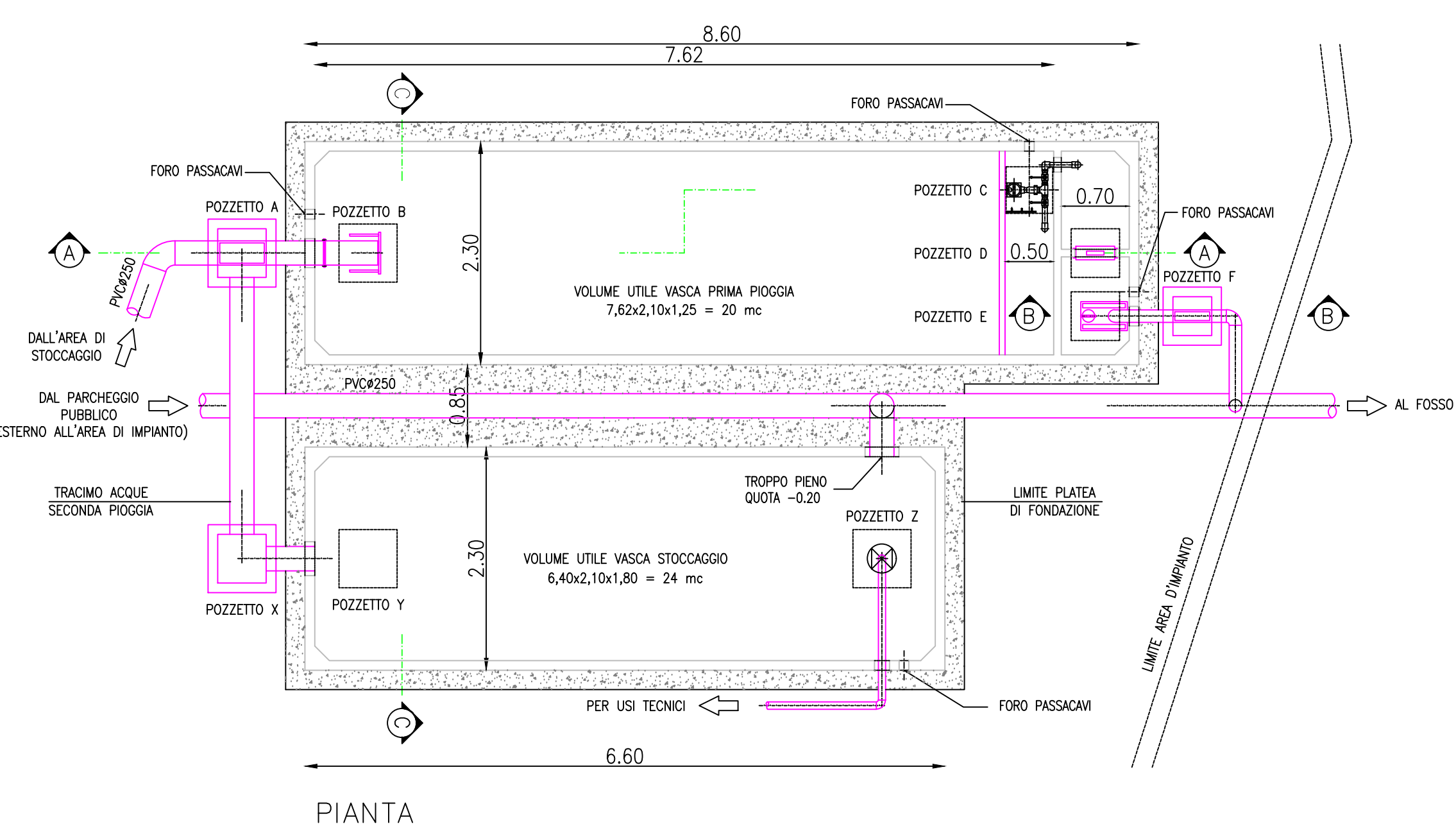
IMPIANTO PRIMA PIOGGIA ESISTENTE 1:50
