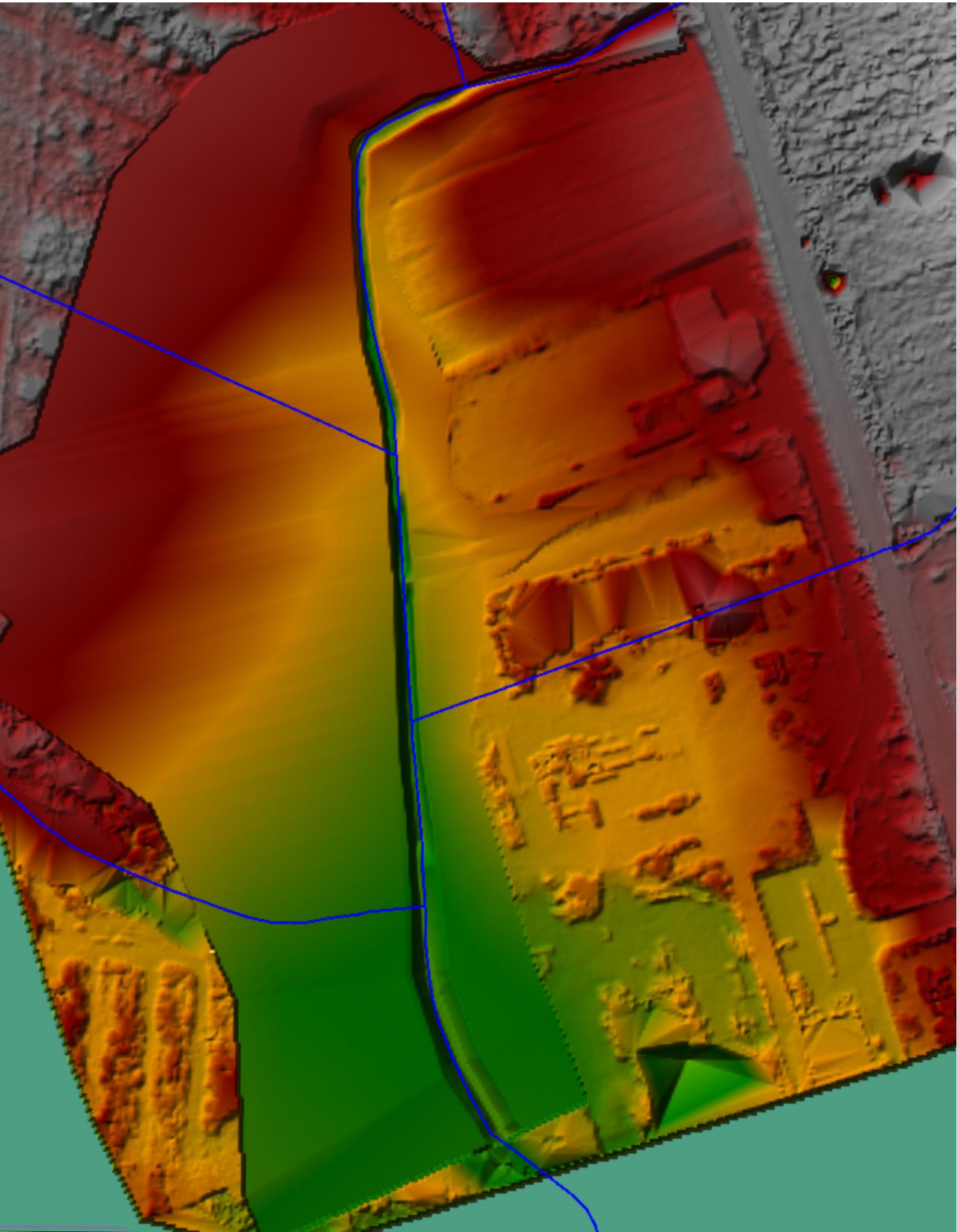
RESTITUZIONE MODELLO 2D - RILIEVO AEROFOTOGRAMMETRICO EFFETTUATO CON DRONE - SCALA 1:500
