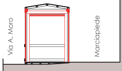
Sezione B-B
