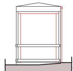
Prospetto nord-est
