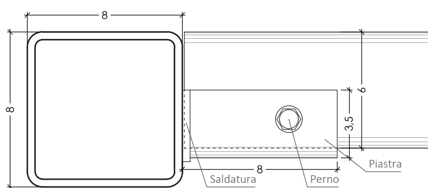
Particolare dell'ancoraggio trave/travetto
