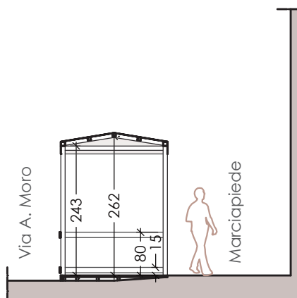
Sezione B-B
