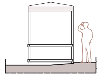
Prospecto nord-est
